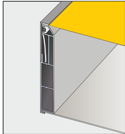
Schnittzeichnung Profil
