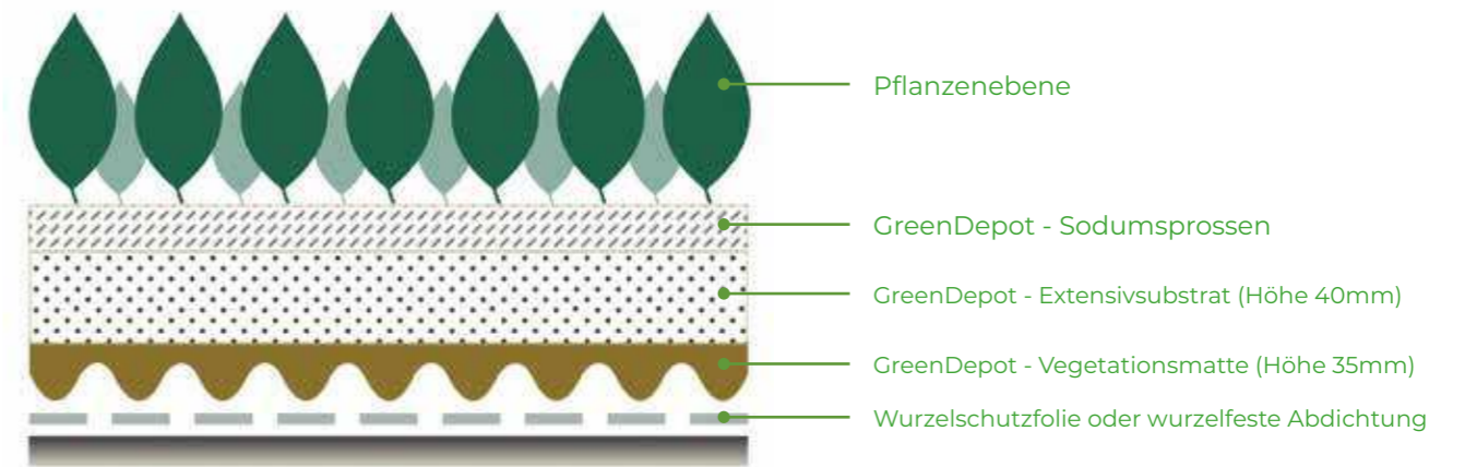
Dachaufbau
